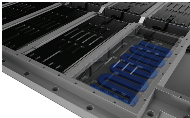
SikaBiresin® TCギャップフィラーを使用したモジュールの熱管理
